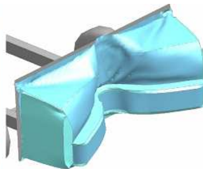
b) Pole test
